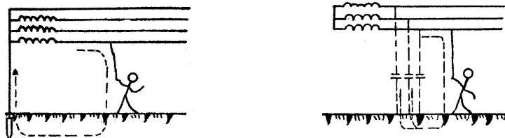
图 2-1 中性点接地系统的单线触电 图 2-2 中性点不接地系统的单线触电
